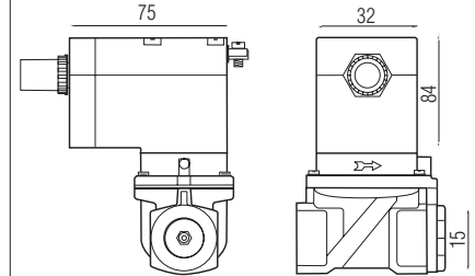
Размеры вентиляльного переходника
